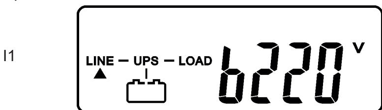
Напряжение на байпасном входе
