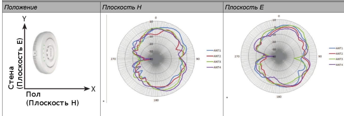
Антенны 5 ГГц при установке на стене
