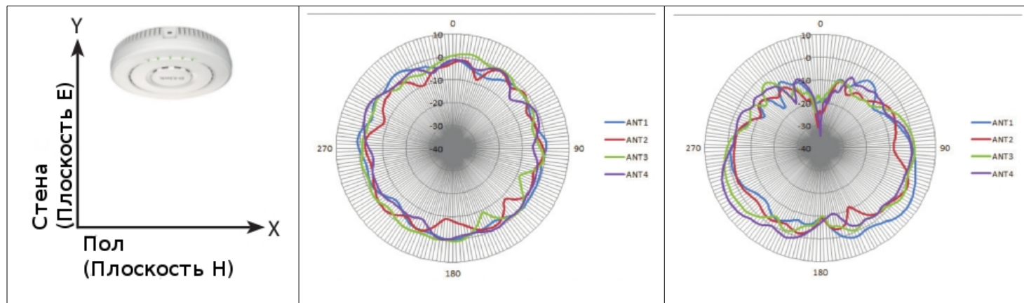
Антенны 5 ГГц при установке на стене
